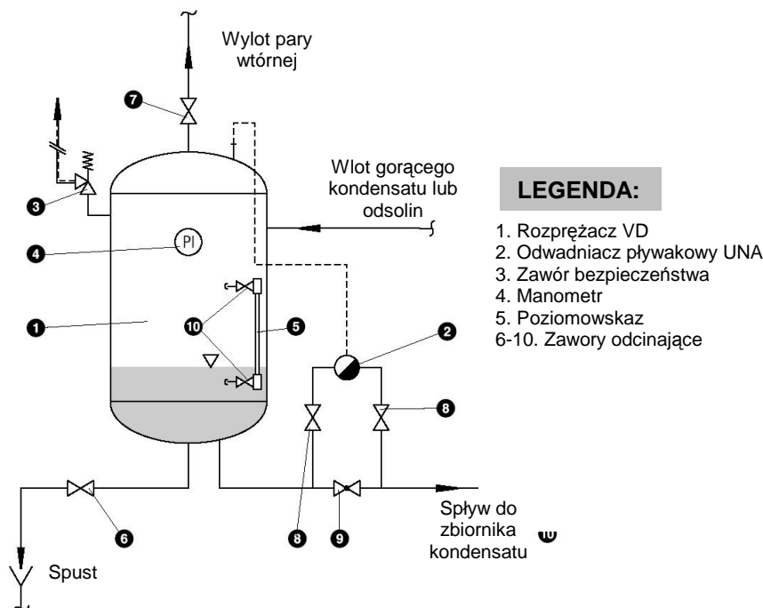
Rys. 2. Schemat ideowy systemu rozprężania
