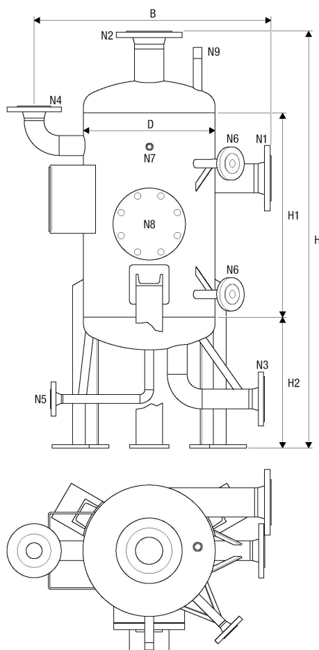
Rys. 3. Szczegóły wymiarowe
