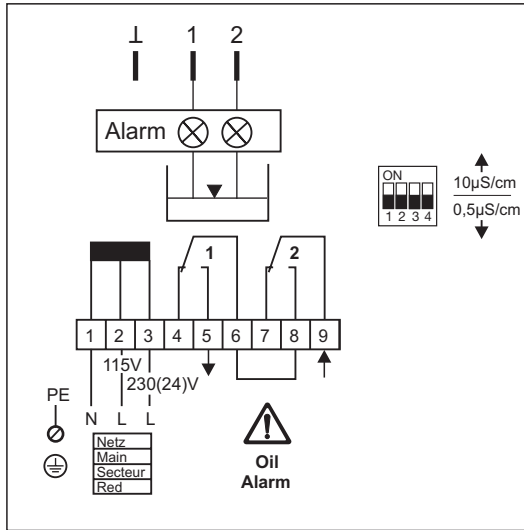
Fig. 8 Dargestellte Kontaktstellung: stromlos, Alarm, LEDs 1 und 2 leuchten nicht!
